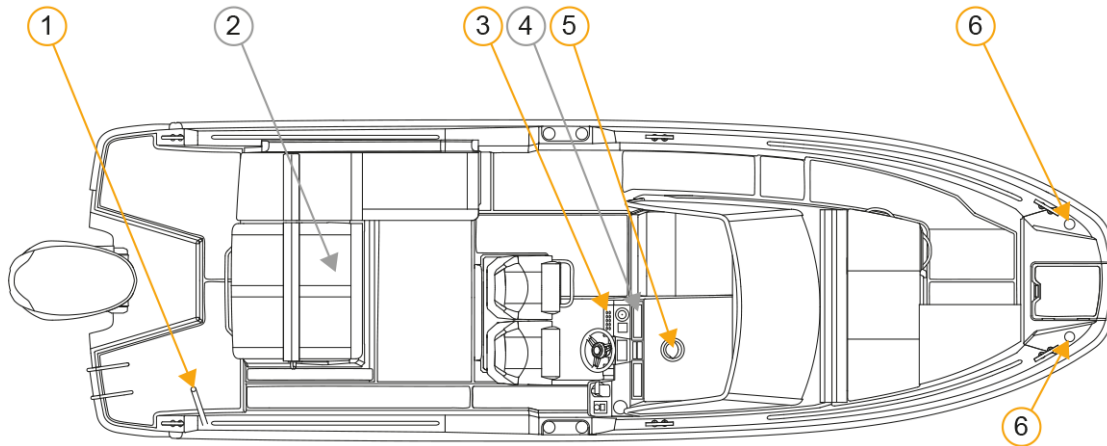
Figur 4.8 Navigationssystemets komponenter
