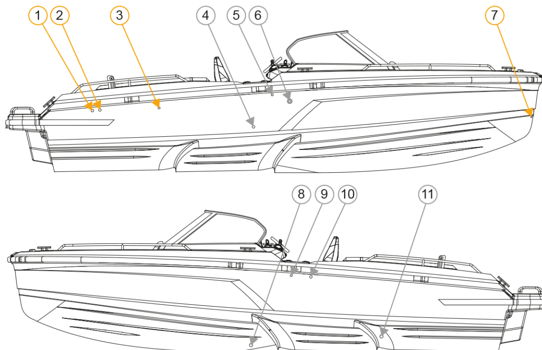
Figur 4.12 Skrovöppningar
