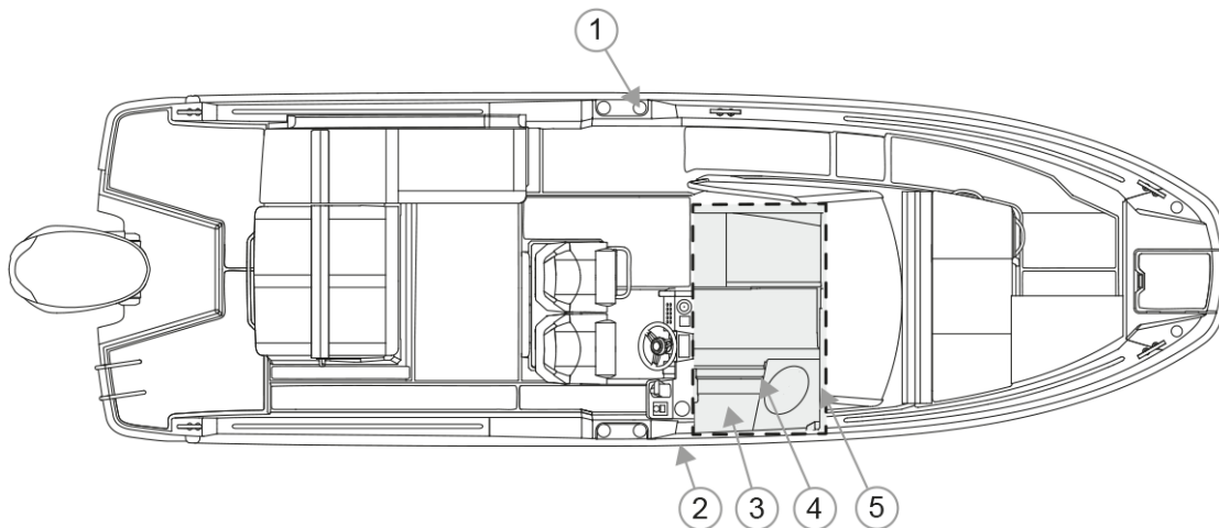
Figur 4.16 Värmarens komponenter
